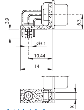
Metallwinkel mit P.o.F. Metal bracket with P.o.F.
